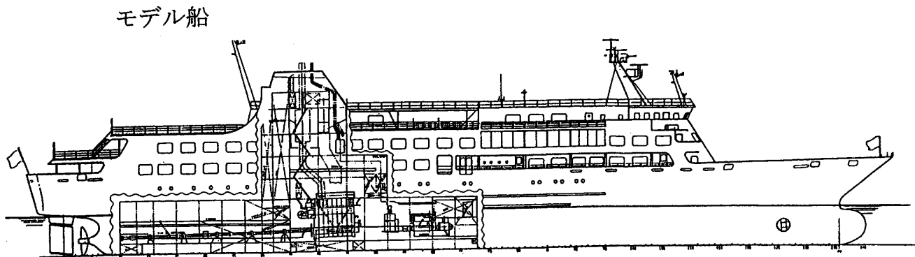
図2 モデル船全体側面図
