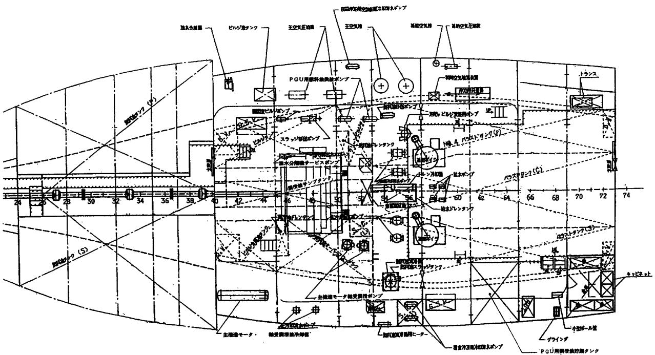
図6 新プラント船の機関室平面図
