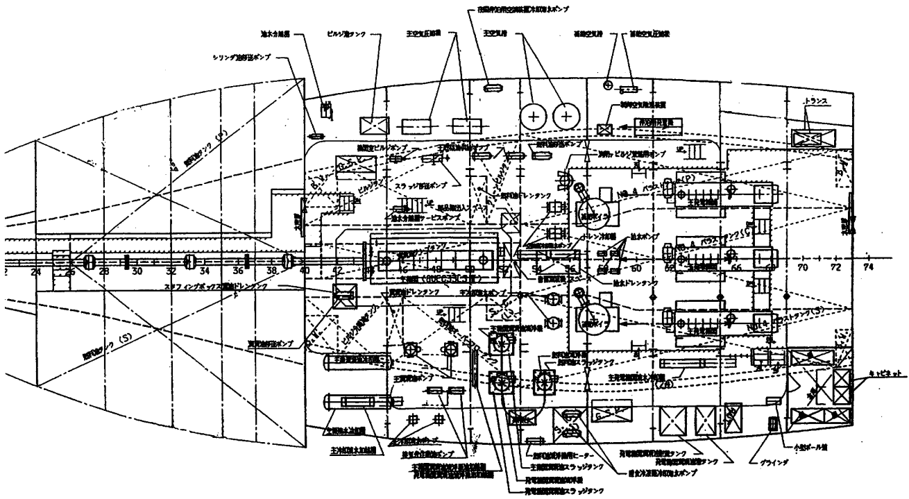
図5 モデル船の機関室平面図
